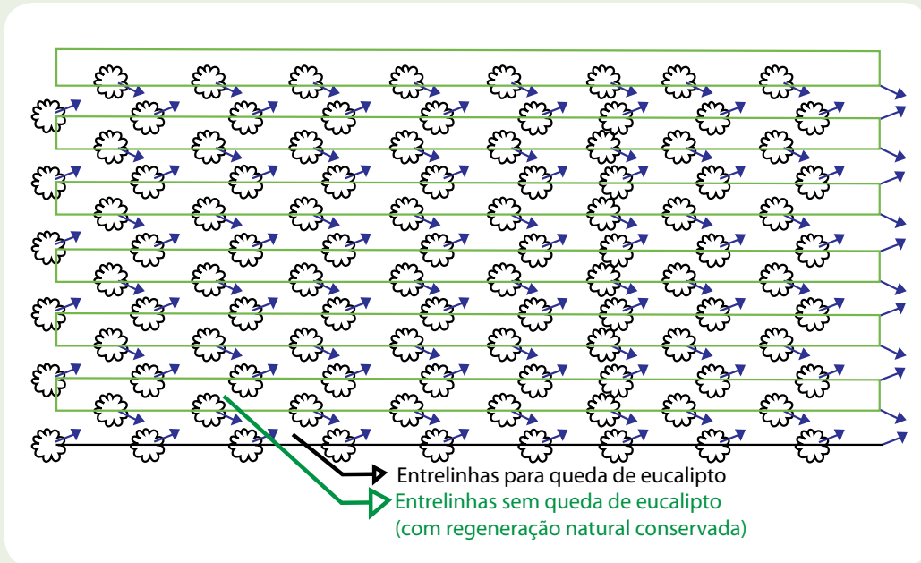
Figura 19 – Esquema de corte de baixo impacto. As setas indicam o sentido da queda dos eucaliptos.
