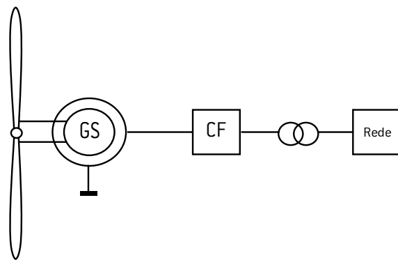
Figura 14 – Aerogerador com gerador síncrono multipolos conectado à rede por conversor de frequência e gerador síncrono
